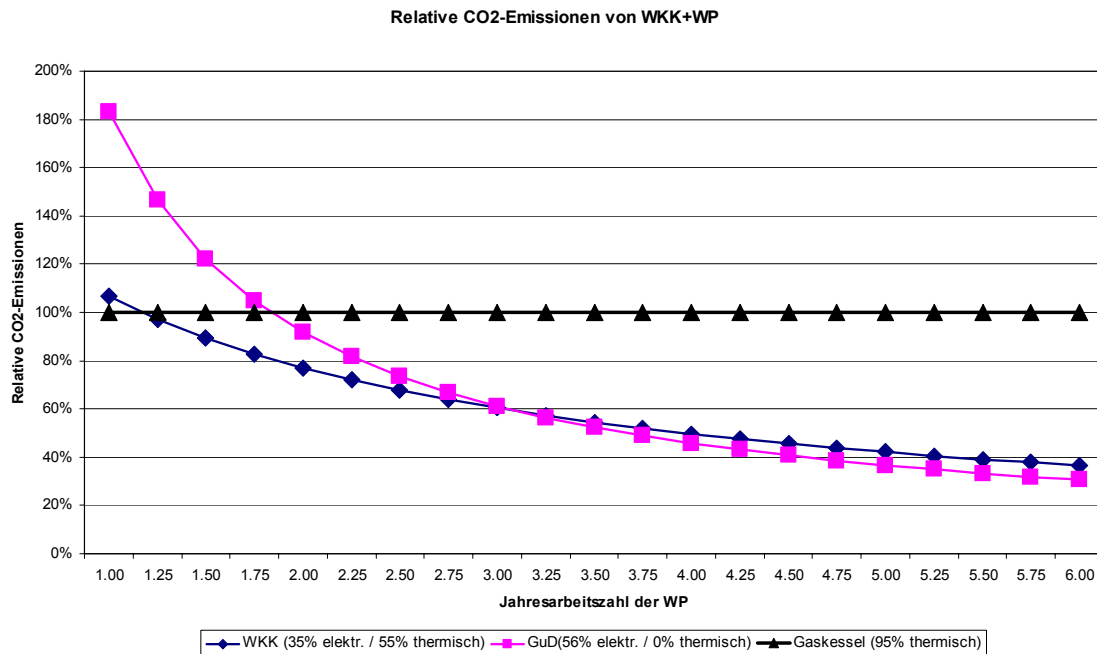
Figur 2: relative CO 2 -Emissionen von Wärmepumpen betrieben mit Strom aus Wärme-Kraft-Kopplung (WKK) oder Gas-Kombi-Kraftwerk (GuD) in Abhängigkeit der Jahresarbeitszahl der Wärmepumpe. Die Prozent-Angaben sind Nutzungsgrade über eine Heizperiode, bezogen auf den unteren Brennwert vom Erdgas. Referenz: Gaskessel kondensierend. Annahmen: Wirkungsgrade der WKK sind 35% elektrisch und 55% thermisch, Wirkungsgrade der GuD sind 56% elektrisch und 0% thermisch (keine Wärmenutzung).
