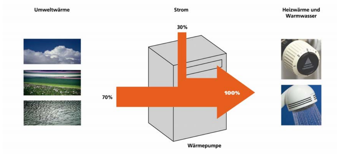
Figur 1: Funktionsprinzip der Wärmepumpe mit Energieflüssen.
